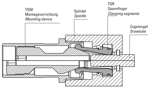
TGM Montagevorrichtung
